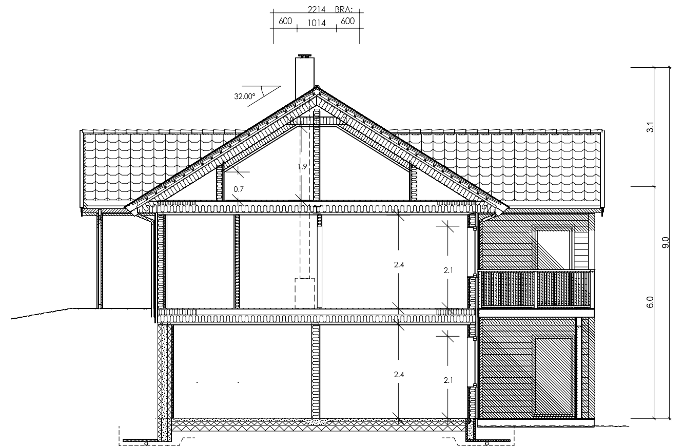
SNITT A-A
