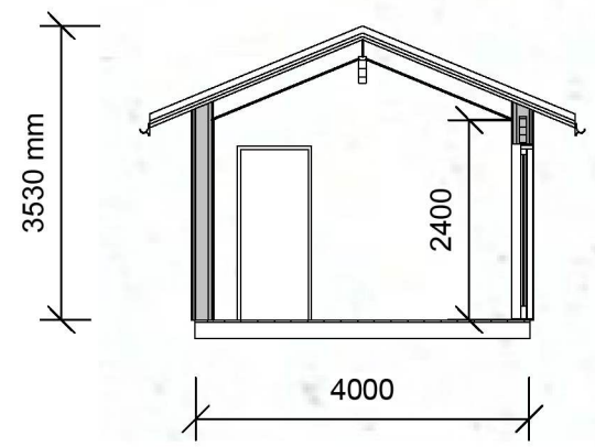
Snitt A
