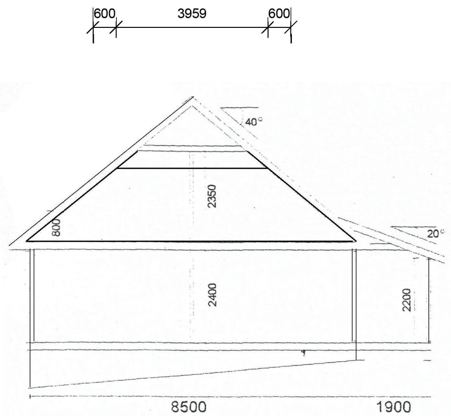
Eksisterende snitt
