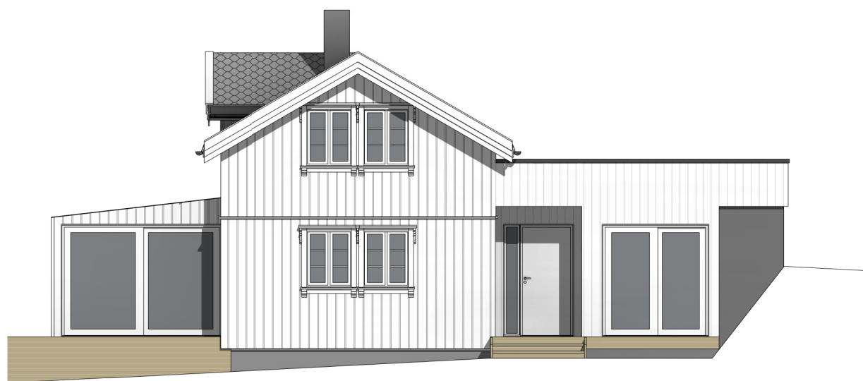
øst 1 : 100
