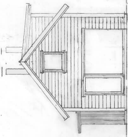
FASADE NORD
