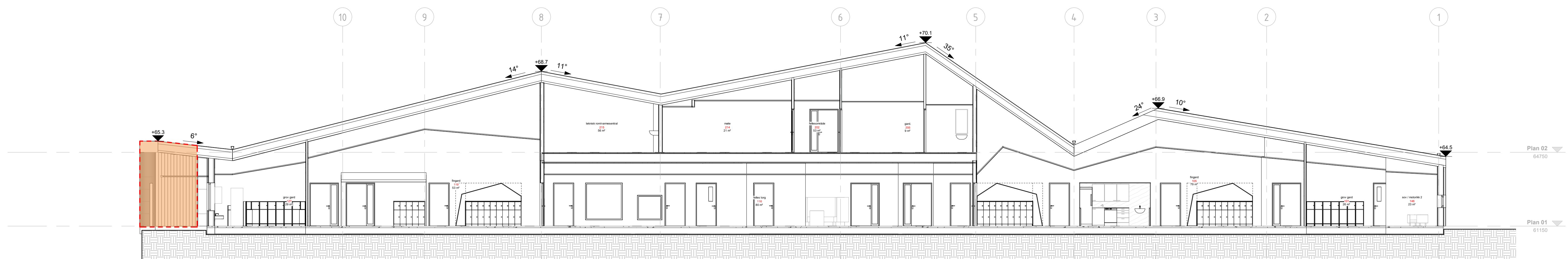
Snitt C-C - endring av tillatelse 1 : 100
