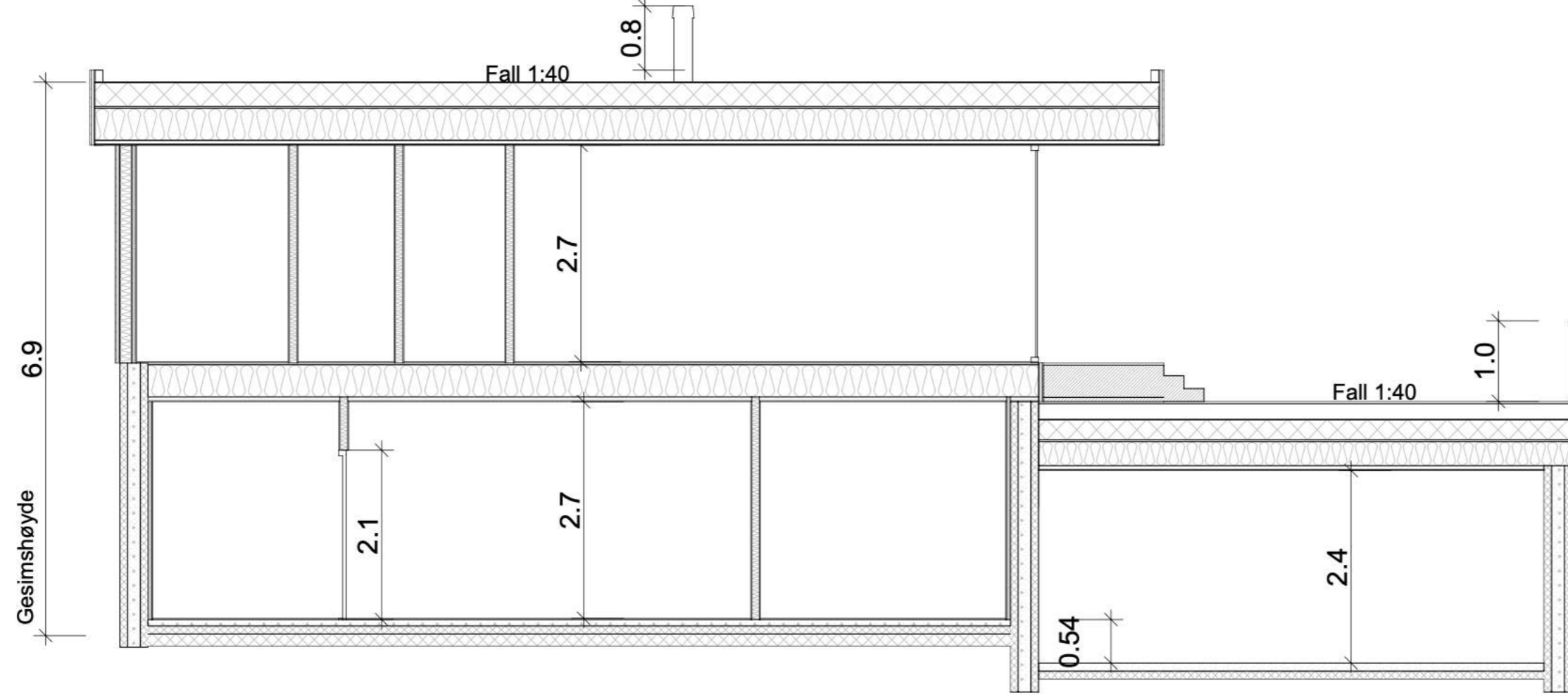
SNITT A-A
