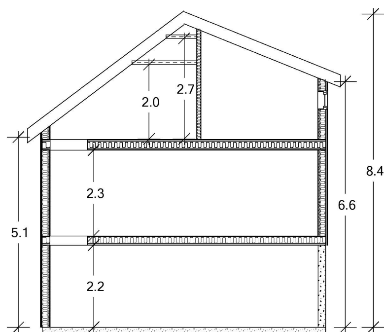
SNITT C-C
