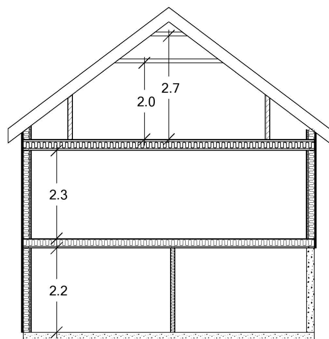
SNITT A-A
