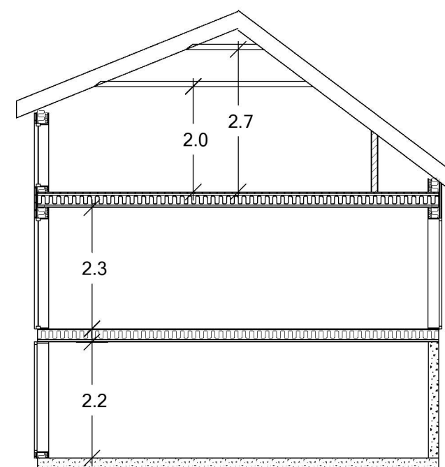
SNITT B-B
