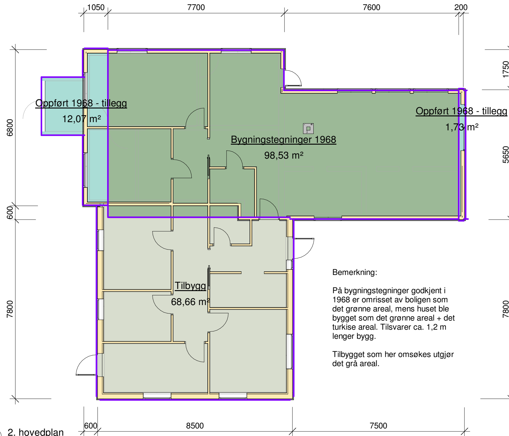
1 2. hovedplan 1 : 100
