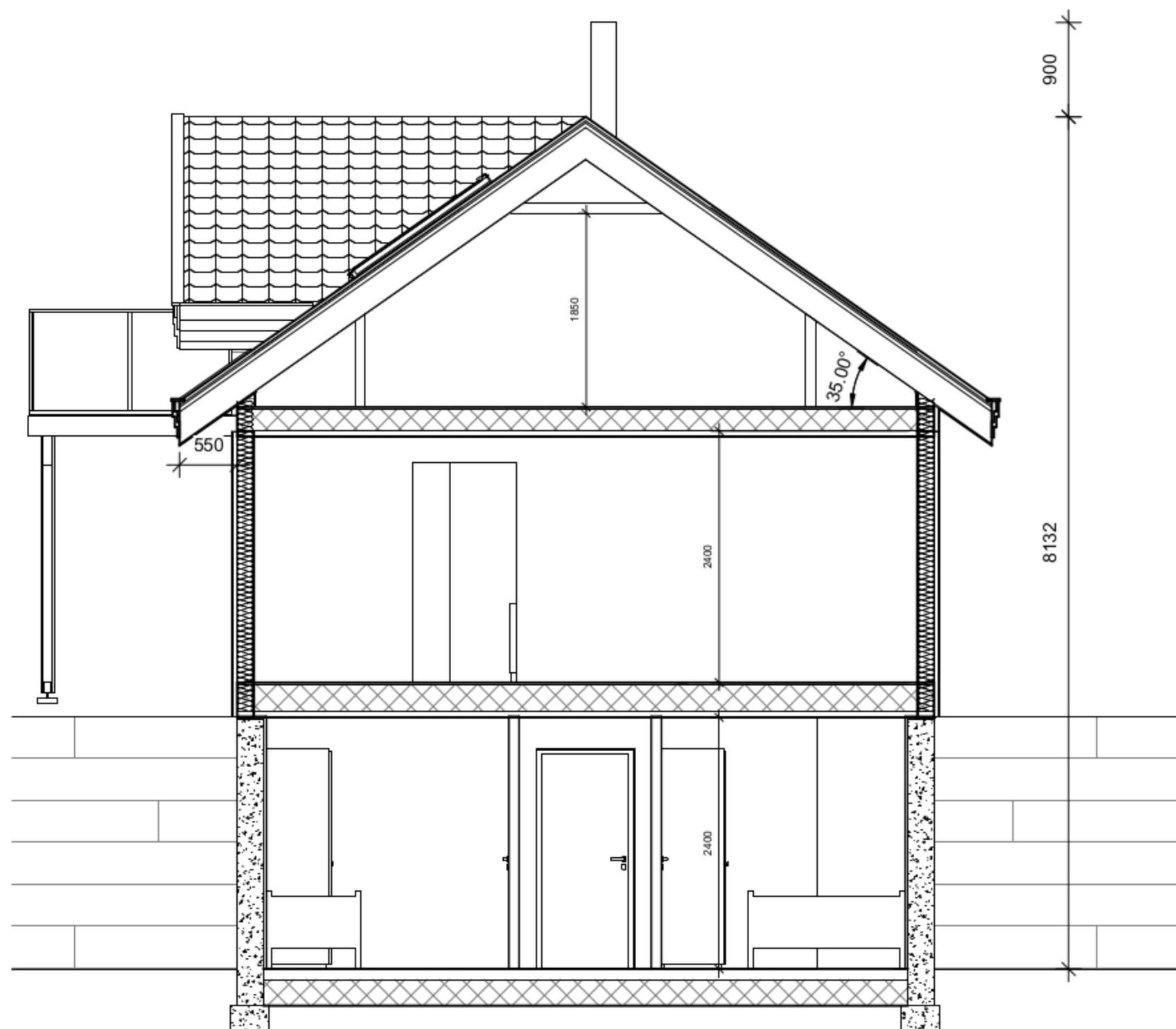
1 Snitt 1 Arb.1-50 1 : 50
