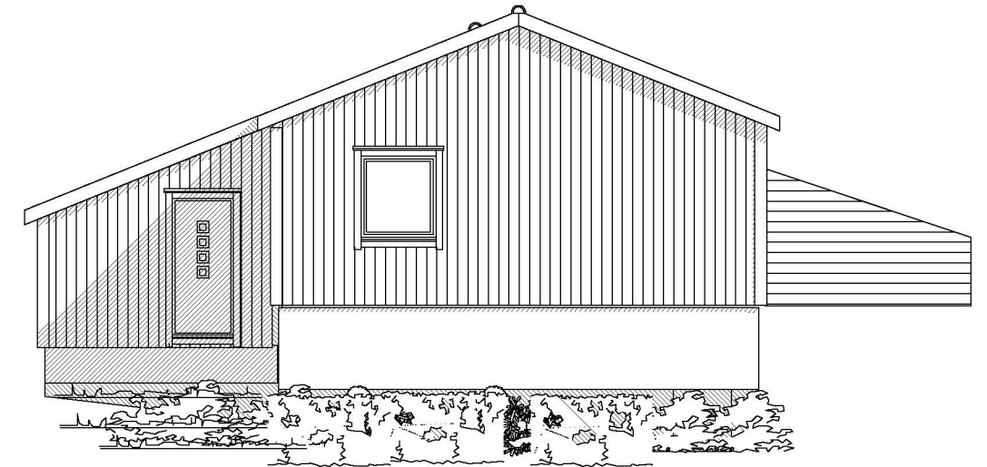
SØR-ØST
