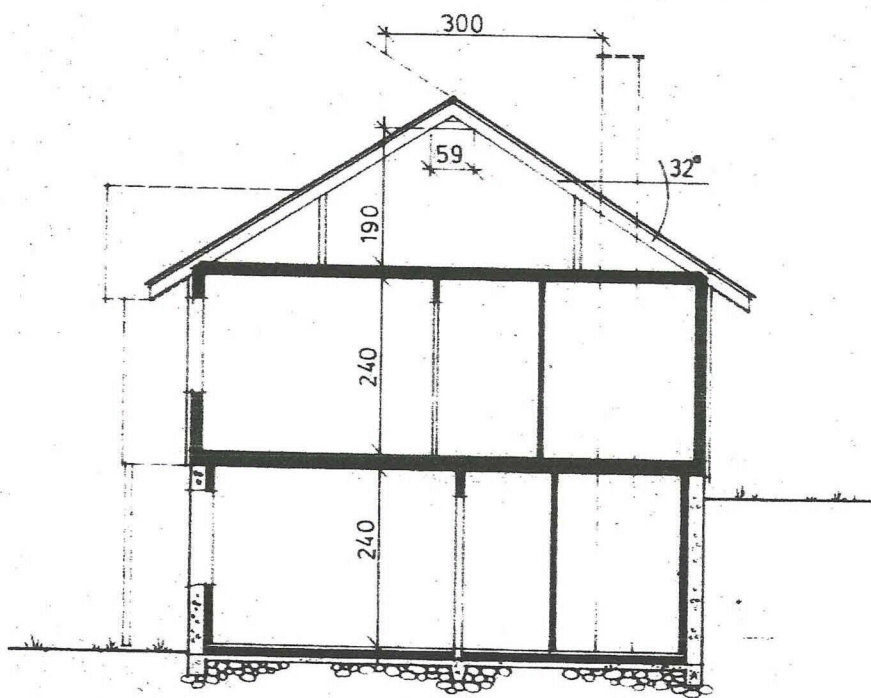
SNITT A-A
