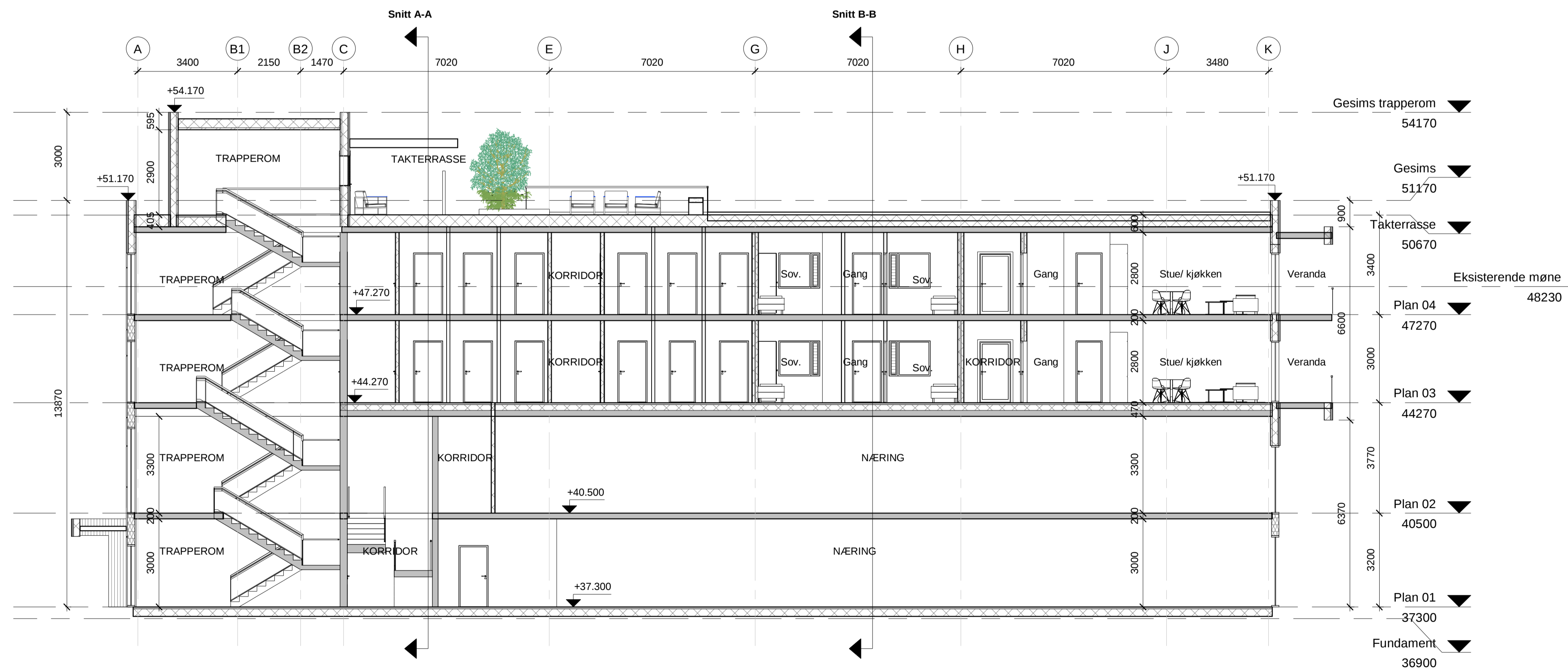
1 Snitt 1-1 1 : 100
