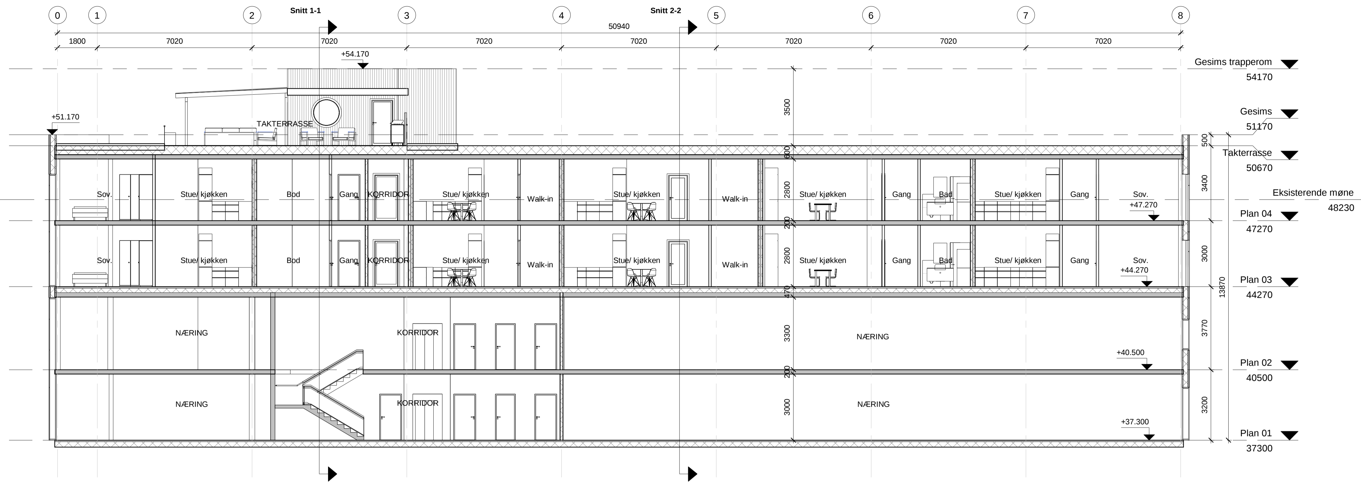
2 Snitt A-A 1 : 100
