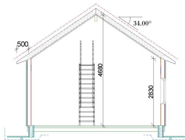
SNITT B-B
