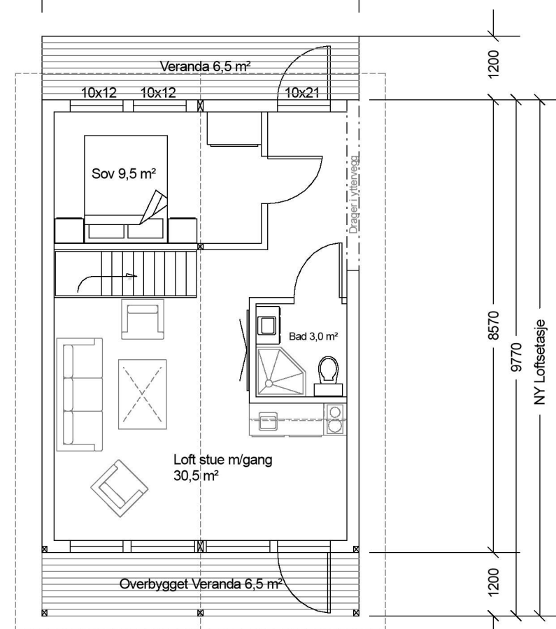
Plantegning loft
