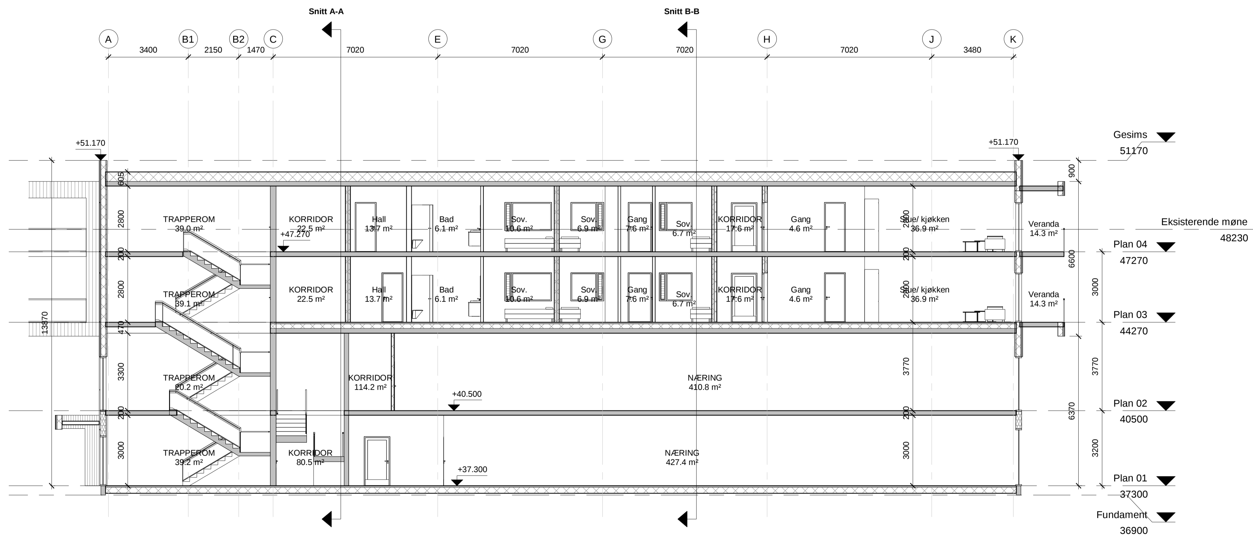
1 Snitt 1-1 1 : 100
