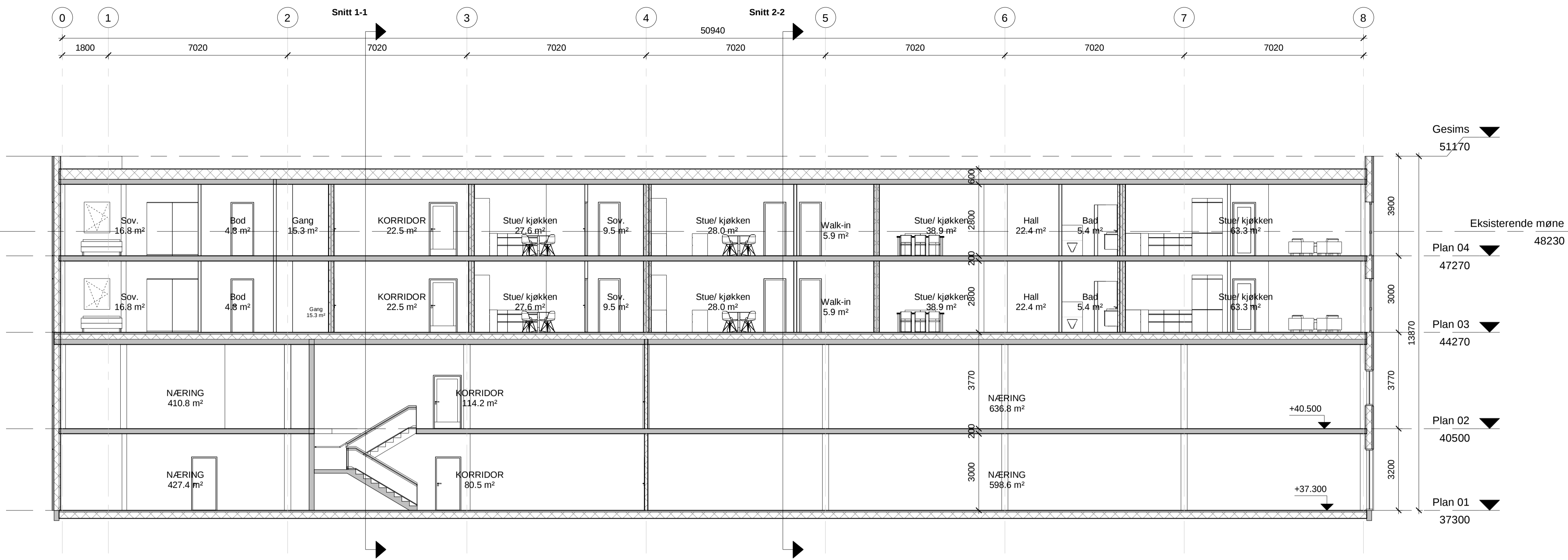
2 Snitt A-A 1 : 100
