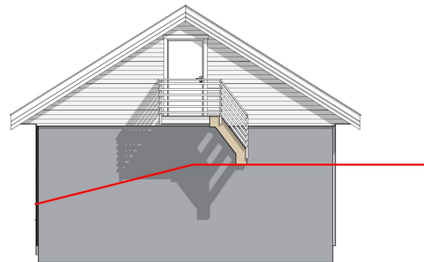
1:100 Fasade Sør
