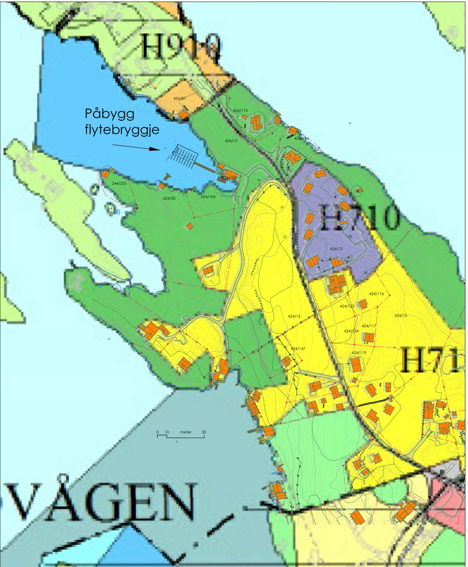
Nordbø 424/13 Påbygg flytebryggje Oversiktskart - med kommuneplankart under 090821 / VM
