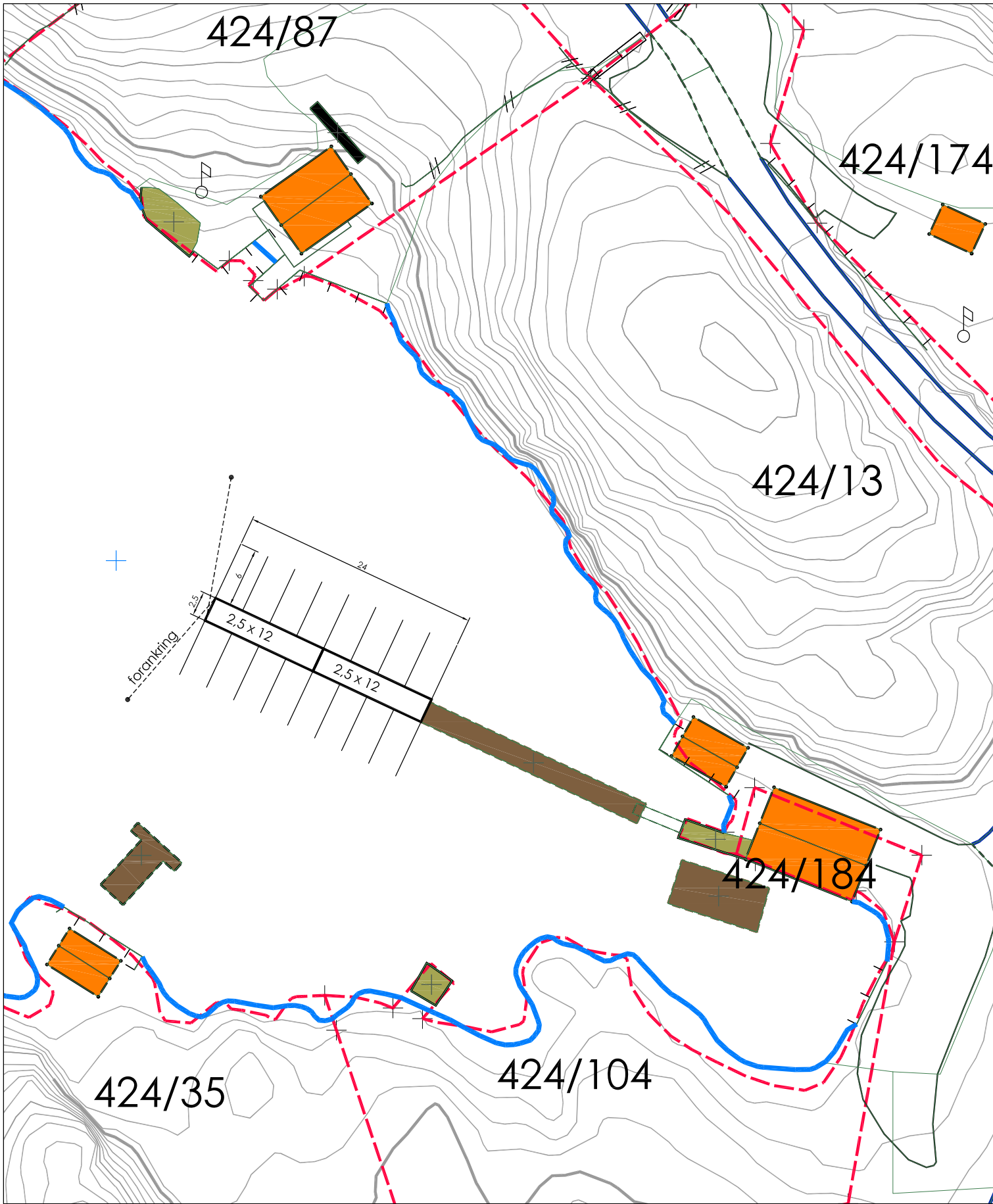
Nordbø 424/13 Påbygg flytebryggje Situasjonsplan 090821 / VM
