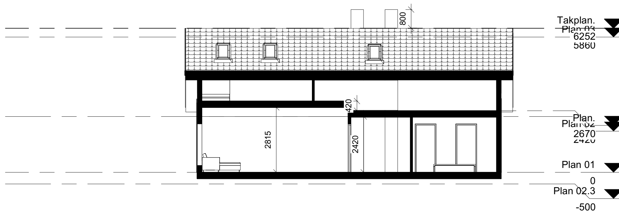
1 SNITT 1 1 : 100
