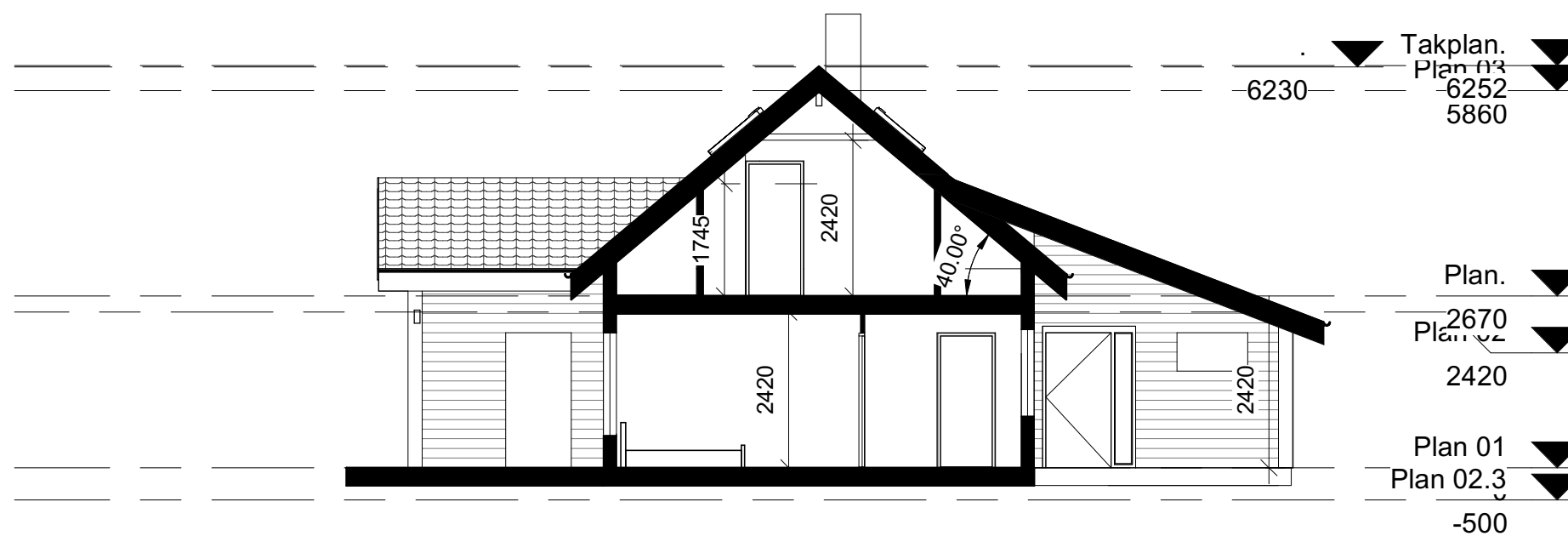
1 SNITT 1 1 : 100
