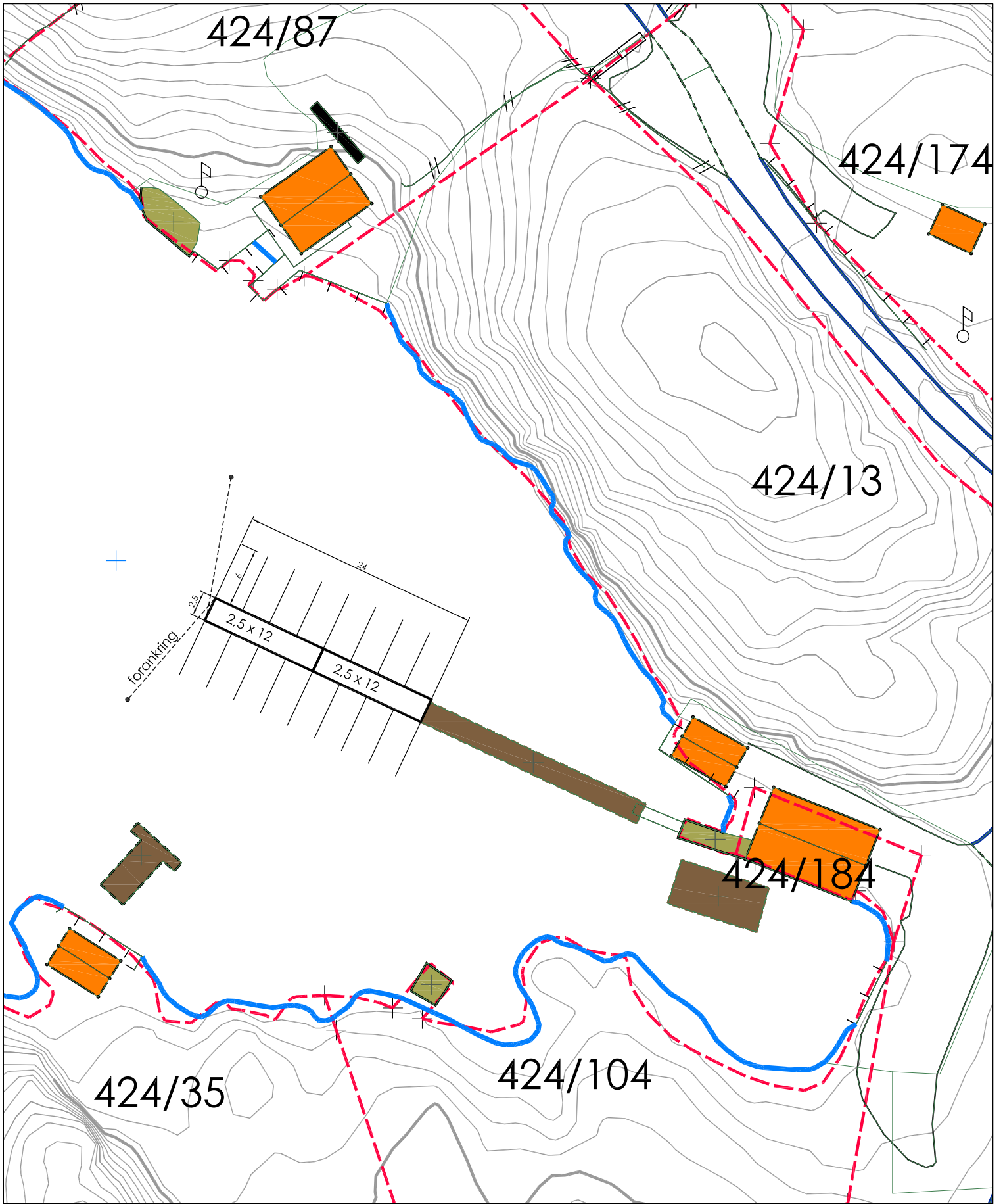
Nordbø 424/13 Påbygg flytebryggje Situasjonsplan 090821 / VM
