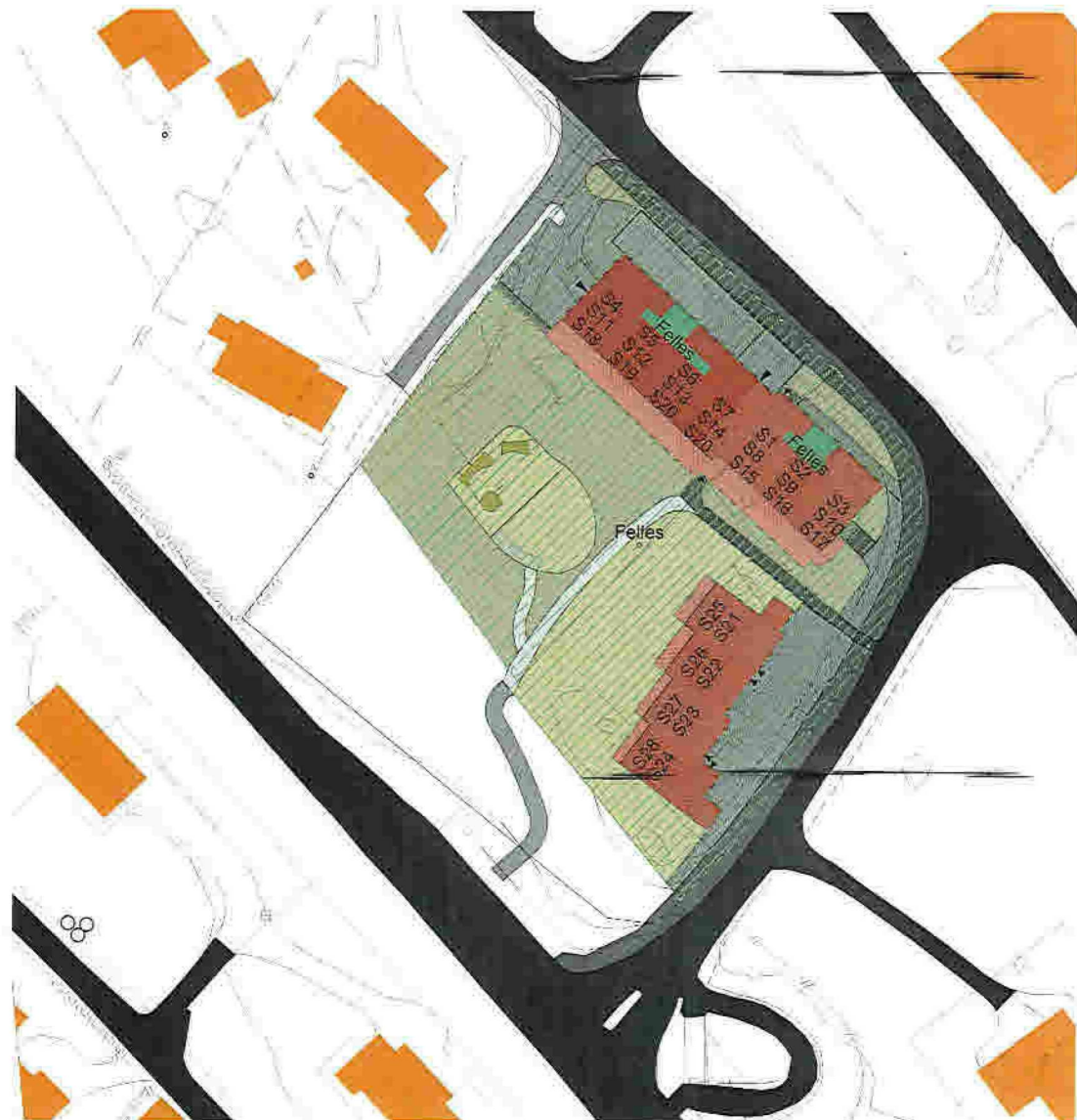
1:500 Situasjonsplan
