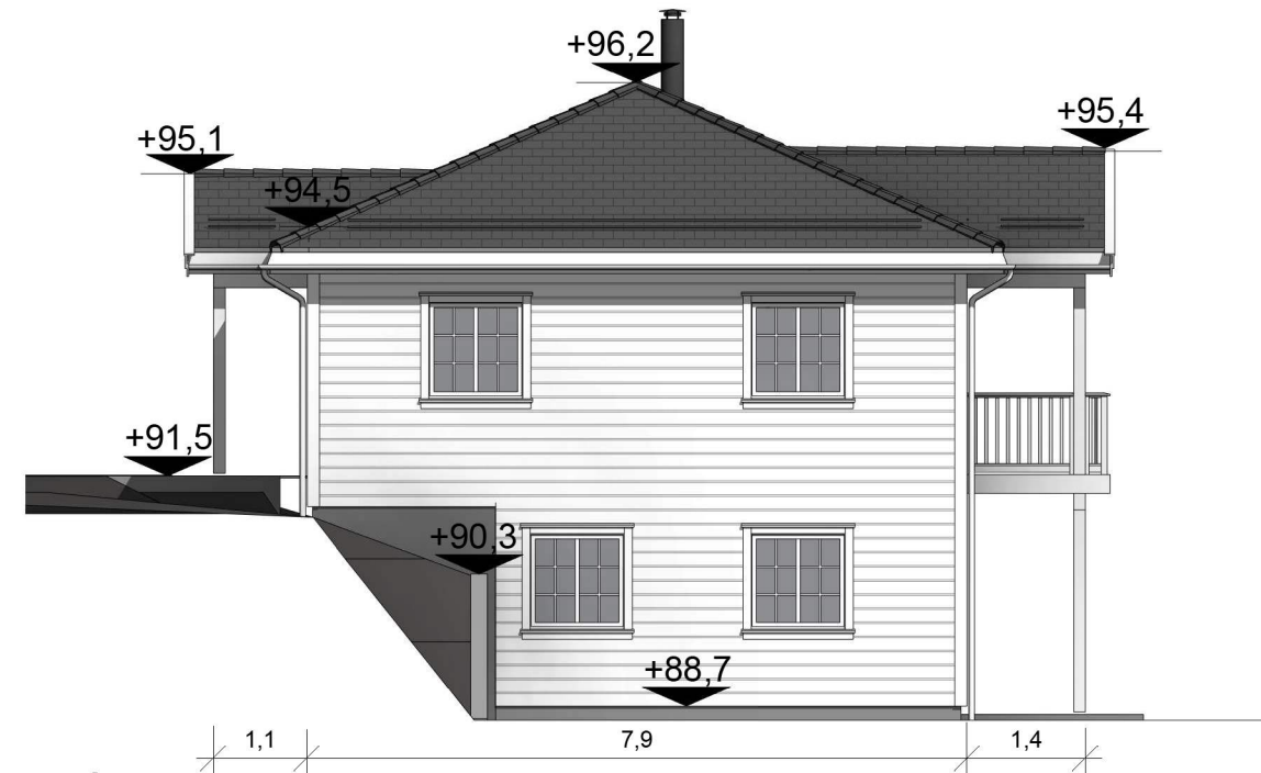
nordvest 1 : 100
