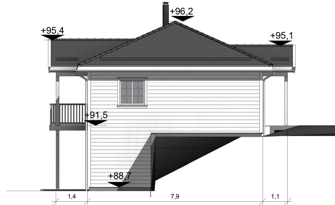
sørøst 1 : 100
