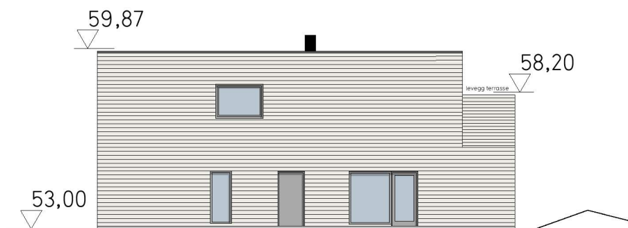
Fasade nord
