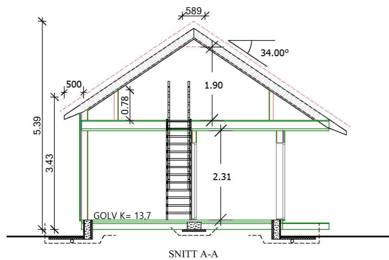
SNITT A-A
