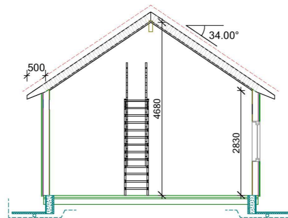
SNITT B-B
