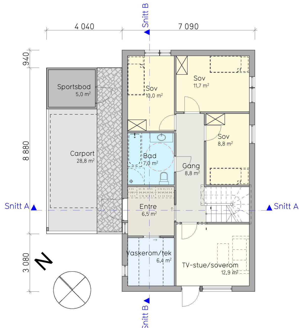
1. etasje
