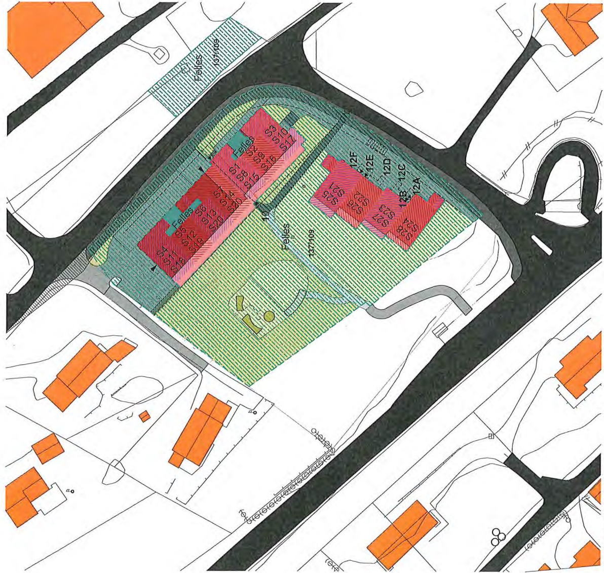
1:500 Situasjonsplan
