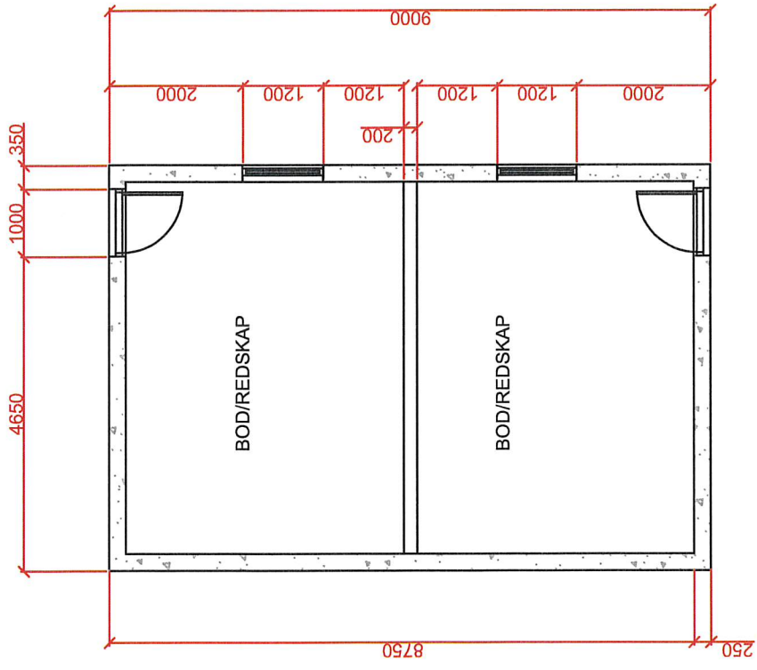
Plan 1.etasje
