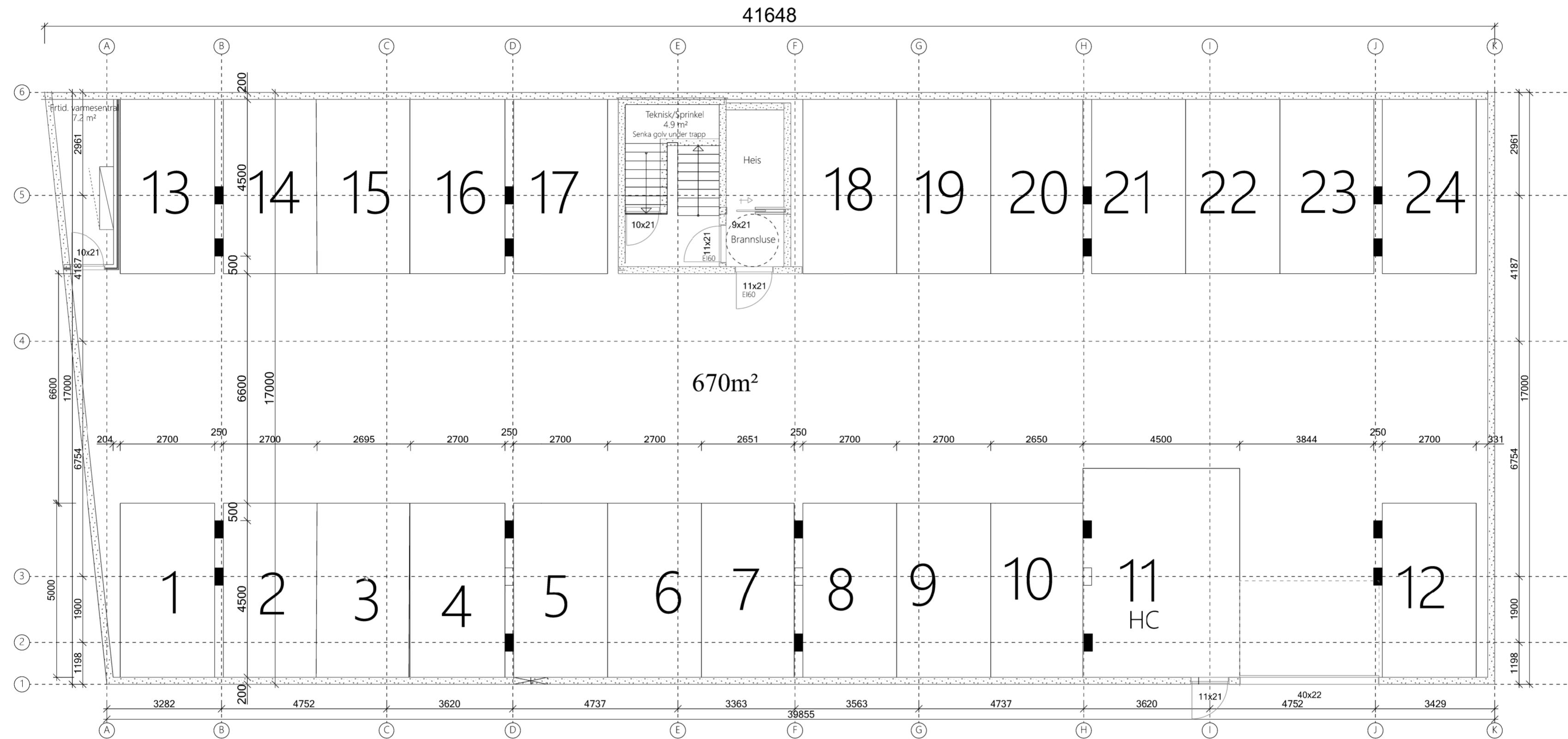
PLAN 0 - Kjellar
