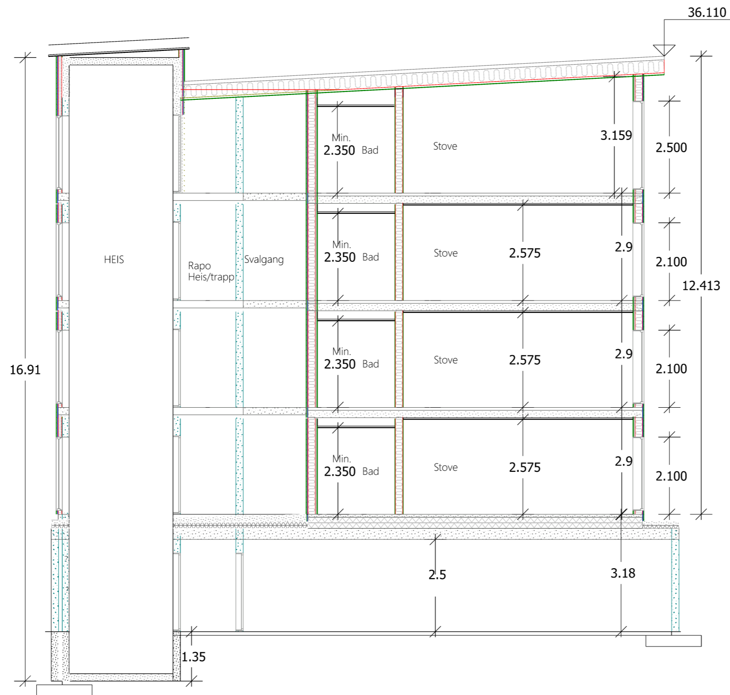
Snitt A-A
