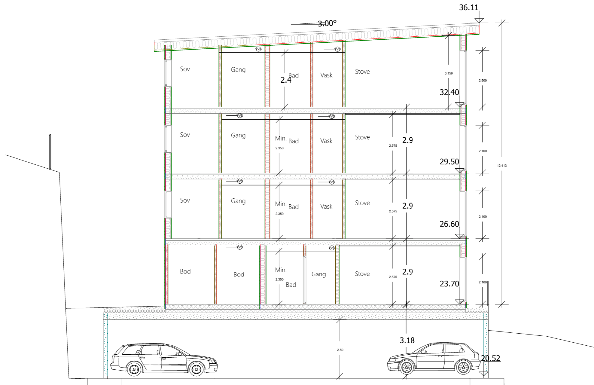
SNITT B-B
