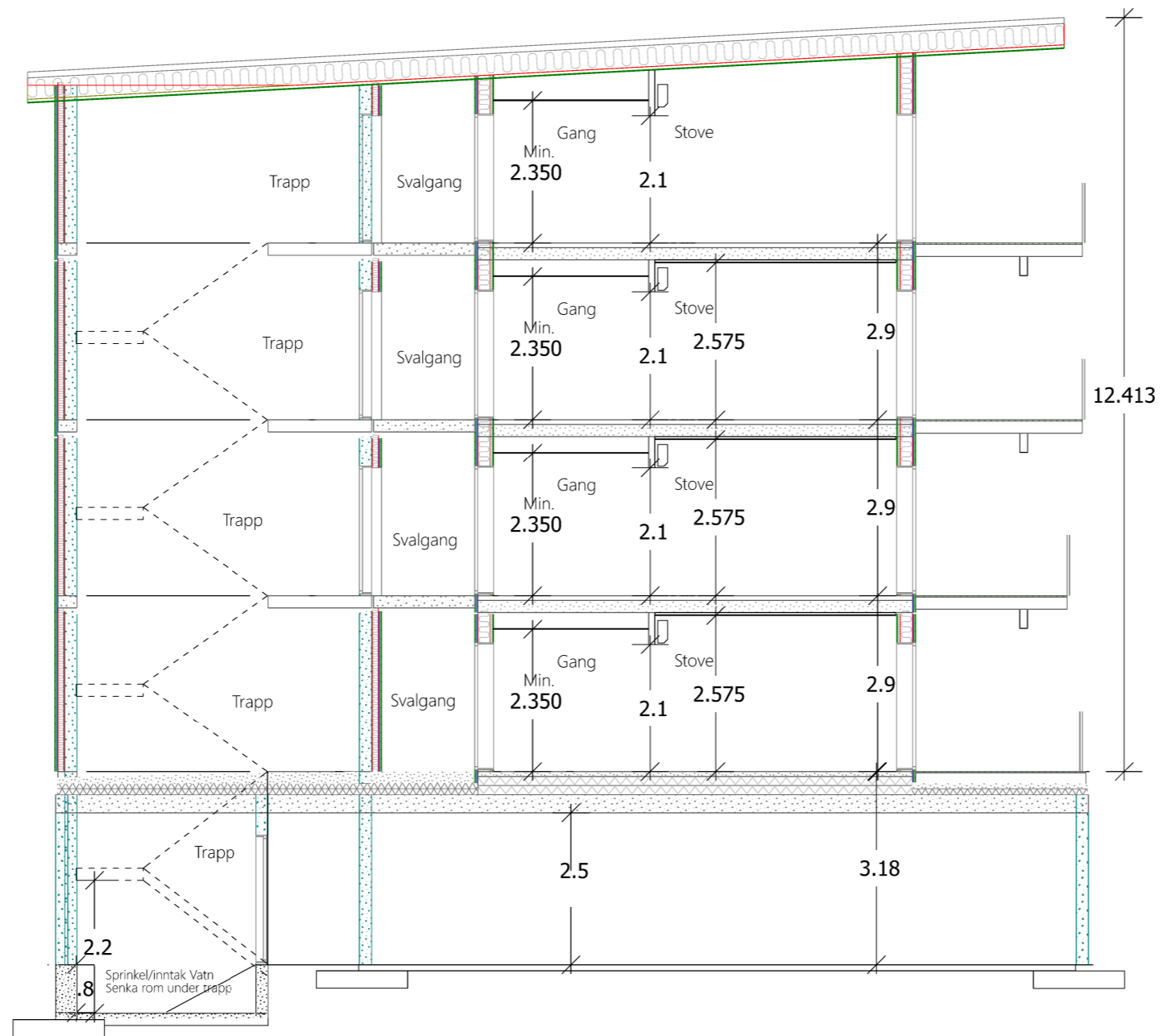
Snitt C-C
