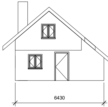
2 North 1 : 100
