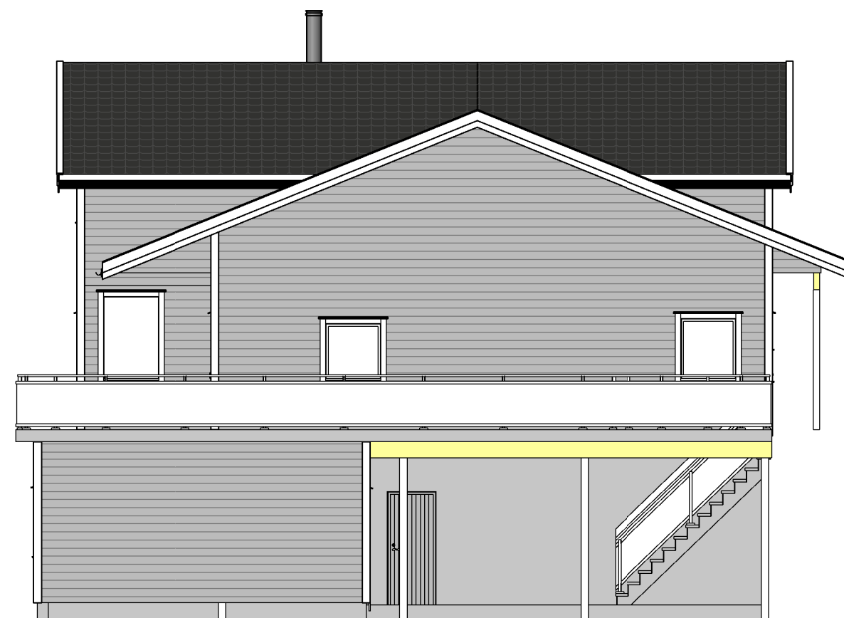
FASADE 4
