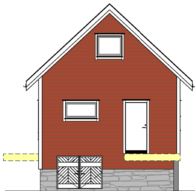
FASADE MOT NORD
