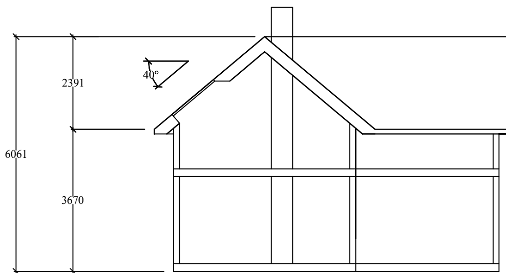
Snitt etter tiltak
