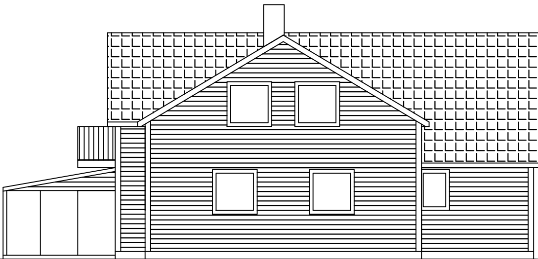
Fasade Øst etter tiltak
