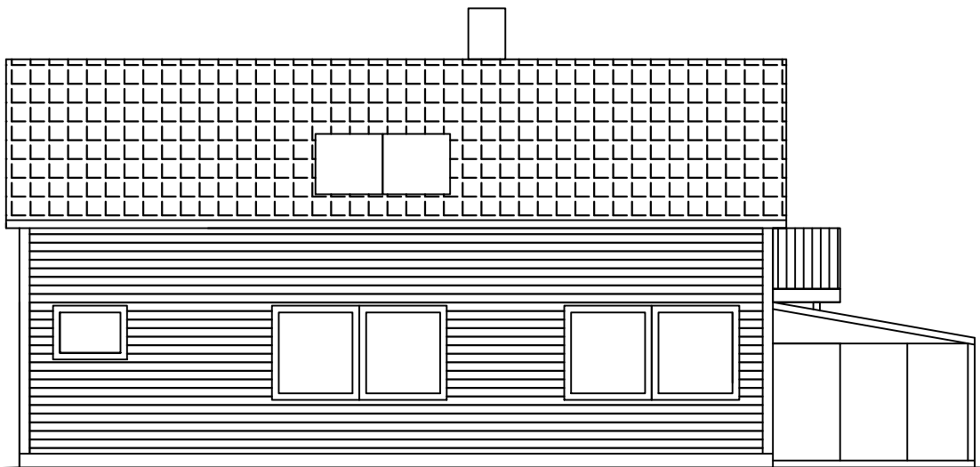
Fasade Vest etter tiltak
