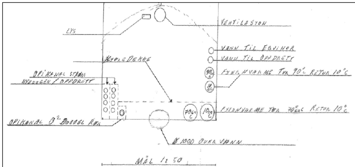
Figur 15: Skisse estimert tversnitt energitunnel. Kjelde: Multiconsult AS.
