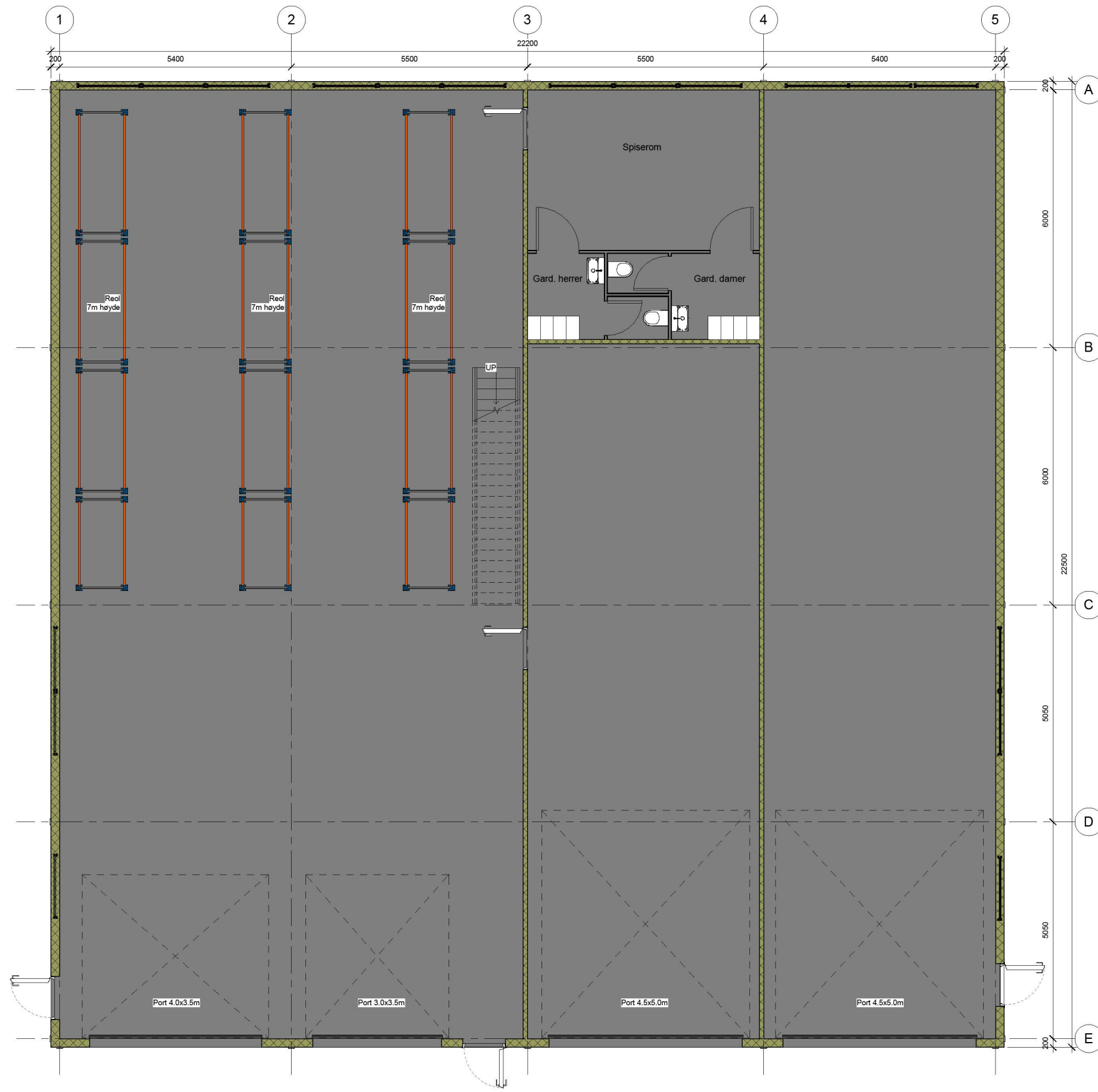
1 Plan 1 1 : 50
