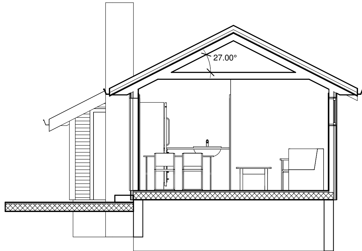
SNITT I STUE
