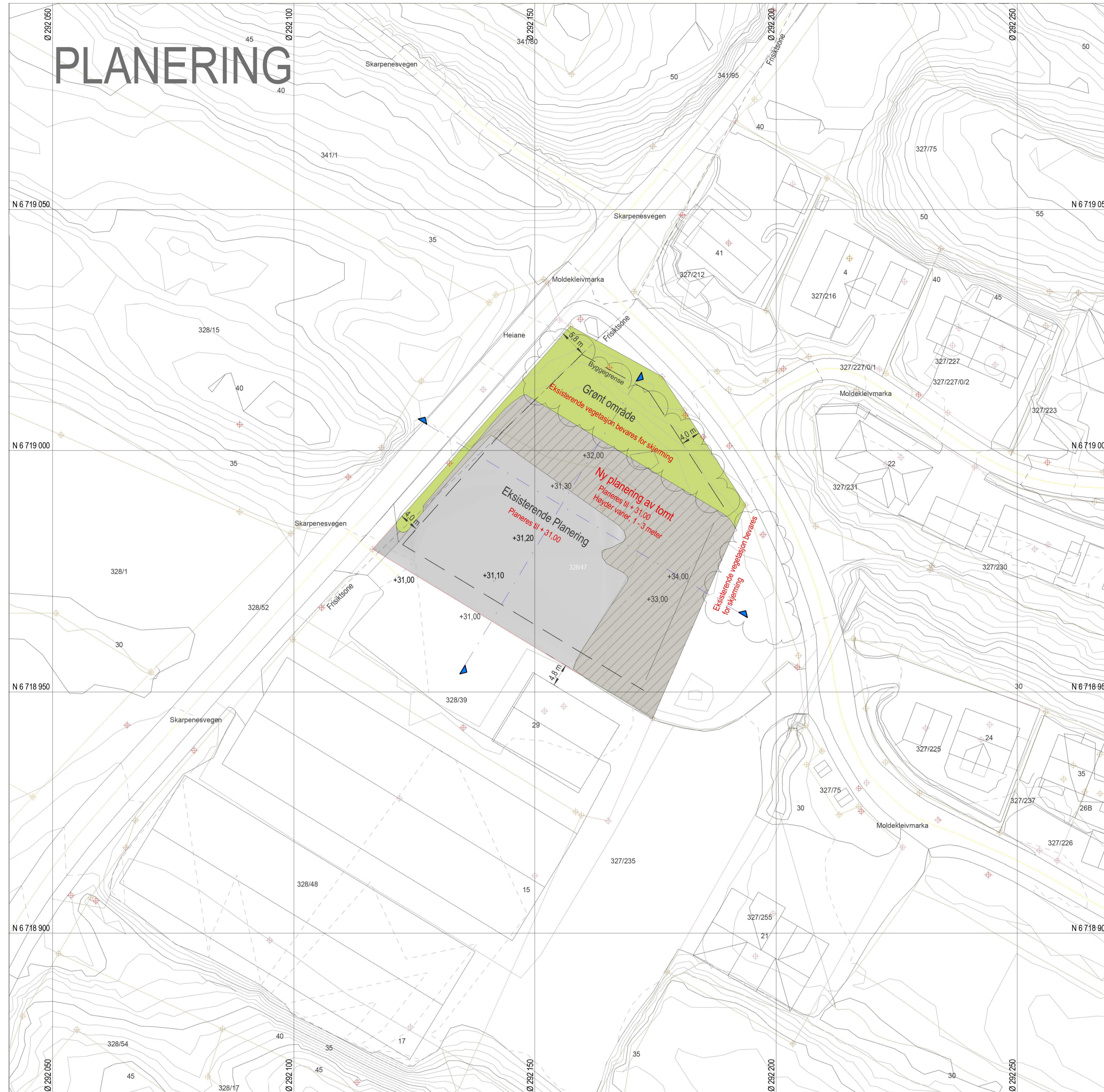
Situasjonsplan - Planering
