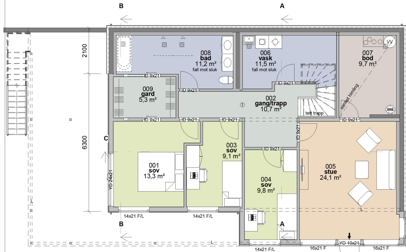
0. Underetasje 1 : 100
