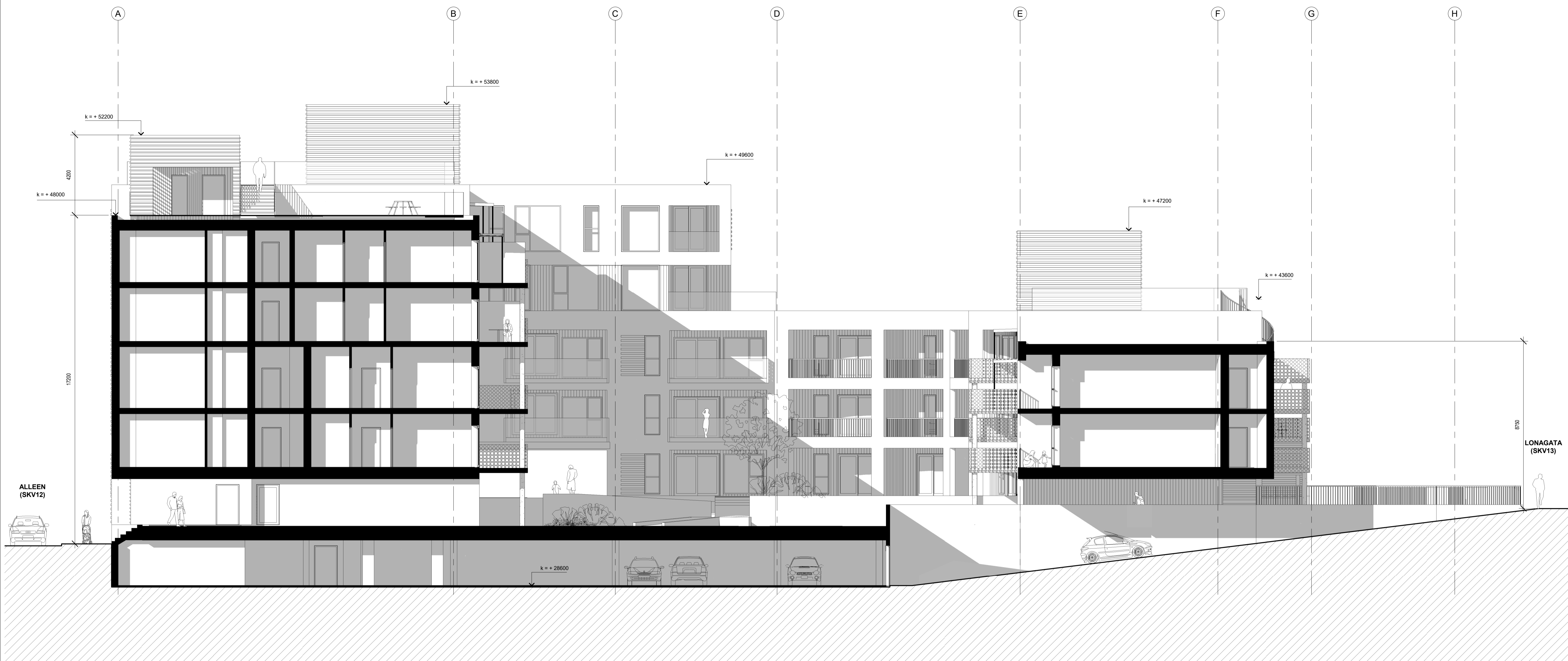
1 Snitt 2-2 1 : 100
