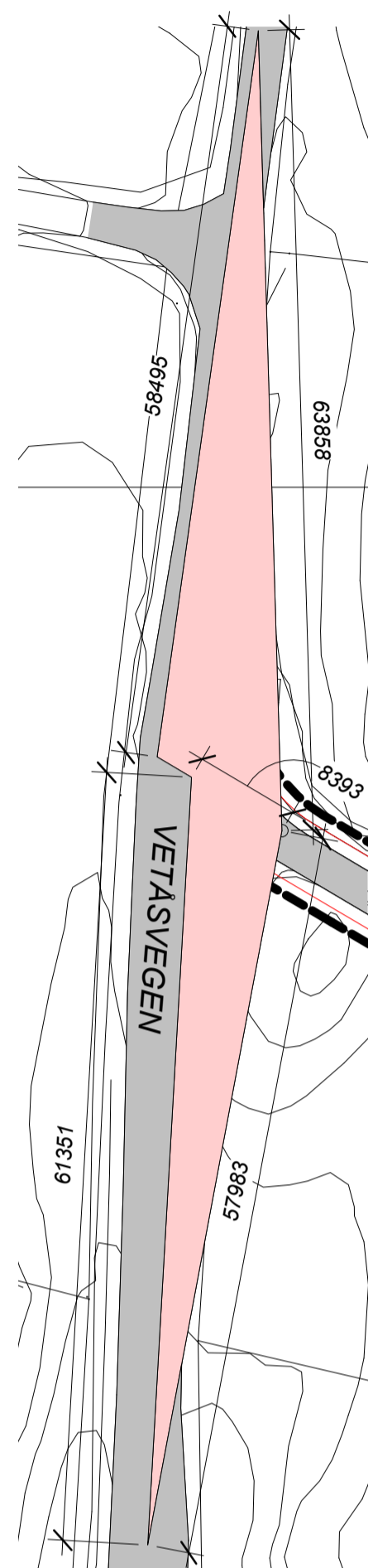
2 Sikotlinjer, avkjørsel 1-500 1 : 500
