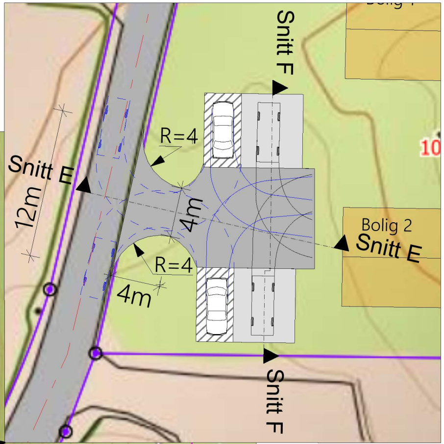
Avkjørselsplan 1:300
