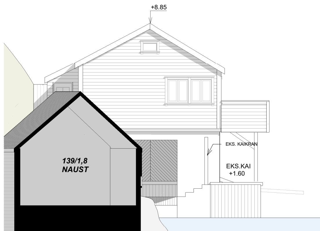
FØR_NØR FASADE_1:100
