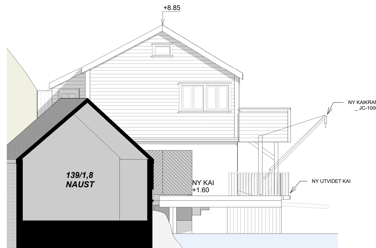
NY_NØR FASADE_1:100
