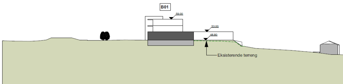
Terrensnitt BB, 1:500
