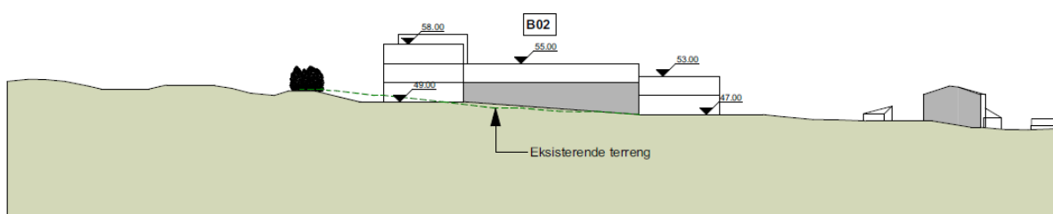
Terrensnitt CC, 1:500
