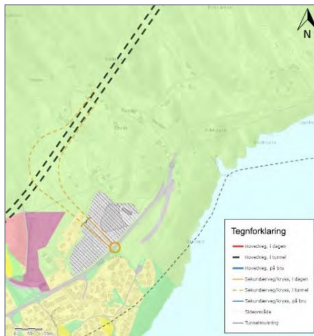
Figur 14. Alternativ V4 vist på arealplan viser kryssing av areal for industri/forretning (grå skravur) i dagsonen i Gjerdvik.
