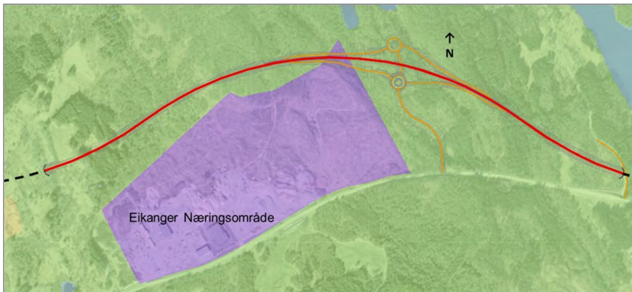
Figur 39. Viser kryssing av område avsatt til næringsvirksomhet (lilla skravor) i Kvernhusdalen for alt. M4.
