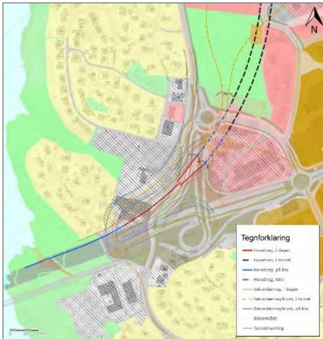
Figur 17. Alternativ V8 vist på arealplan viser kryssing av areal for kontor/industri (grå skravur) i dagsonen i Knarvik.
