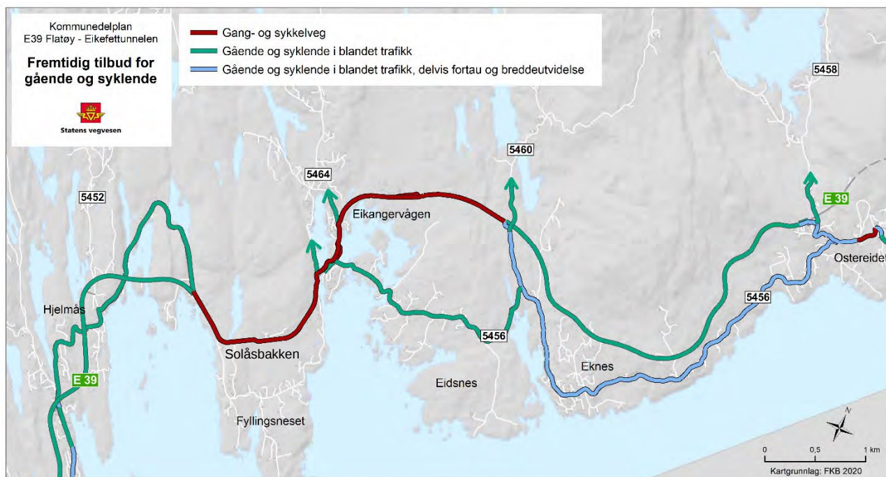
Figur 45. Oversiktstegning fra midtre del av planområdet med forslag til plassering av gang- og sykkelveger.
