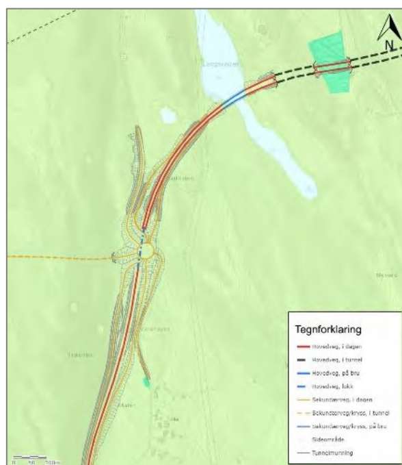
Figur 16. Alternativ V7C vist på arealplan viser kryssing og behov for fylling i LNRF-område/areal med spredt næringsbebyggelse (klar grønn skravur).
