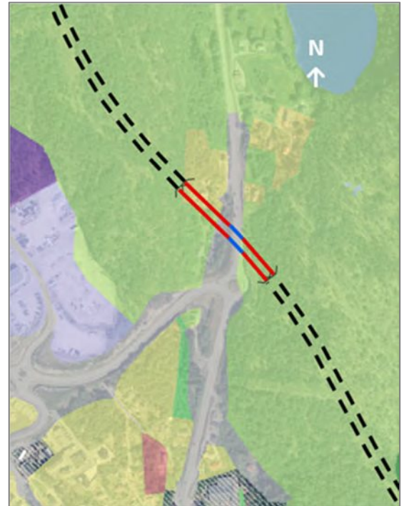
Figur 20. Alternativ V101 vist på arealplan viser kryssing i LNRF-område/areal med tiltak for stedbunden næring (lys grønn skravur) ved dagsonen i Isdal.
