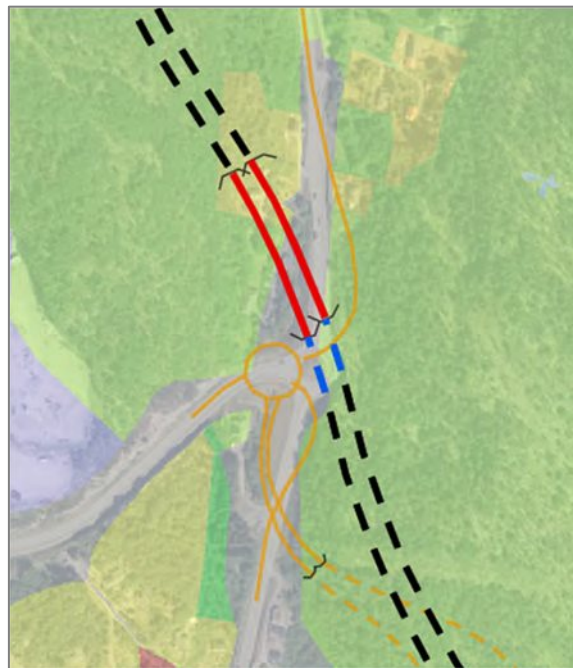
Figur 23. Alternativ V102 vist på arealplan viser kryssing i LNRF-område/areal med tiltak for stedbunden næring (grønn skravur). Sekundærveg krysser boligbebyggelse (lys gul).
