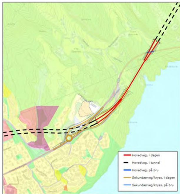
Figur 12. Alternativ V3 vist på arealplan viser kryssing av areal for industri/forretning (grå skravur) i dagsonen i Gjerdvik.
