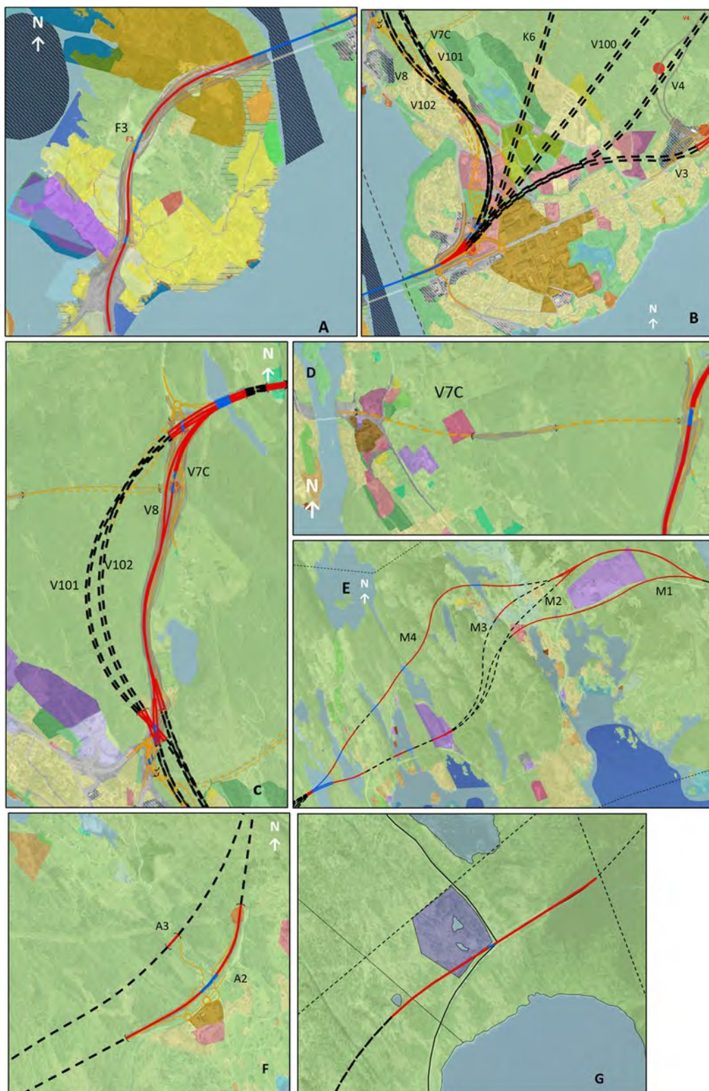
Figur 3. Kartutsnitt av planområdet som viser gjeldende kommune- og kommunedelplaner med nåværende og fremtidige arealformål, samt hovedveglinjer og sekundærveger for de ulike alternative vegtraséene. Rød linje indikerer hovedveg i dagen, blå linje indikerer bru, og stiplet svart linje indikerer hovedveg i tunnel. Merking A-F viser til lokalisering som vist i Figur 2. Fargene for arealformål er også forklart i Figur 2.
