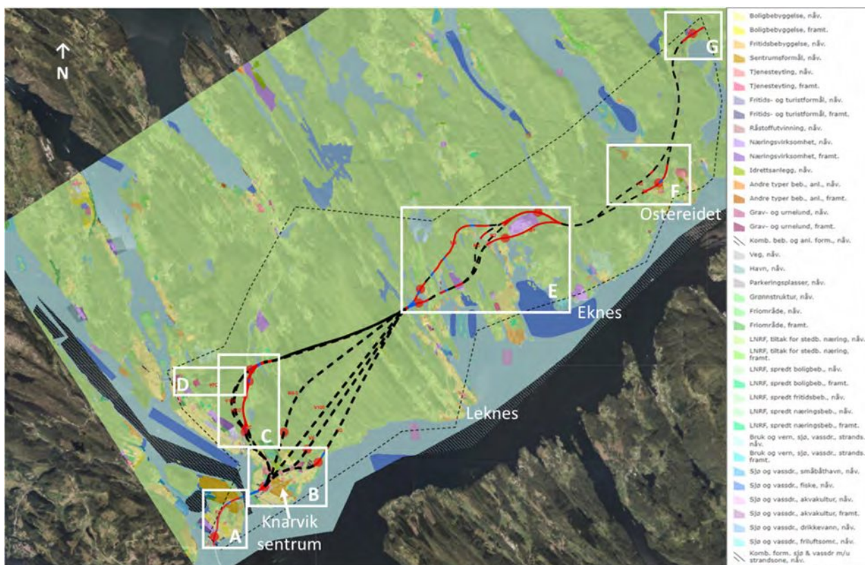
Figur 2. Oversikt over gjeldende kommune- og kommunedelplaner i studieområdet merket med hovedveglinjer for de ulike vegalternativene. Rød linje indikerer hovedveg i dagen, blå linje indikerer bru, rød sirkel viser kryss og stiplet svart linje indikerer hovedveg i tunnel. Utsnitt A til G er videre vist i Figur 3.
