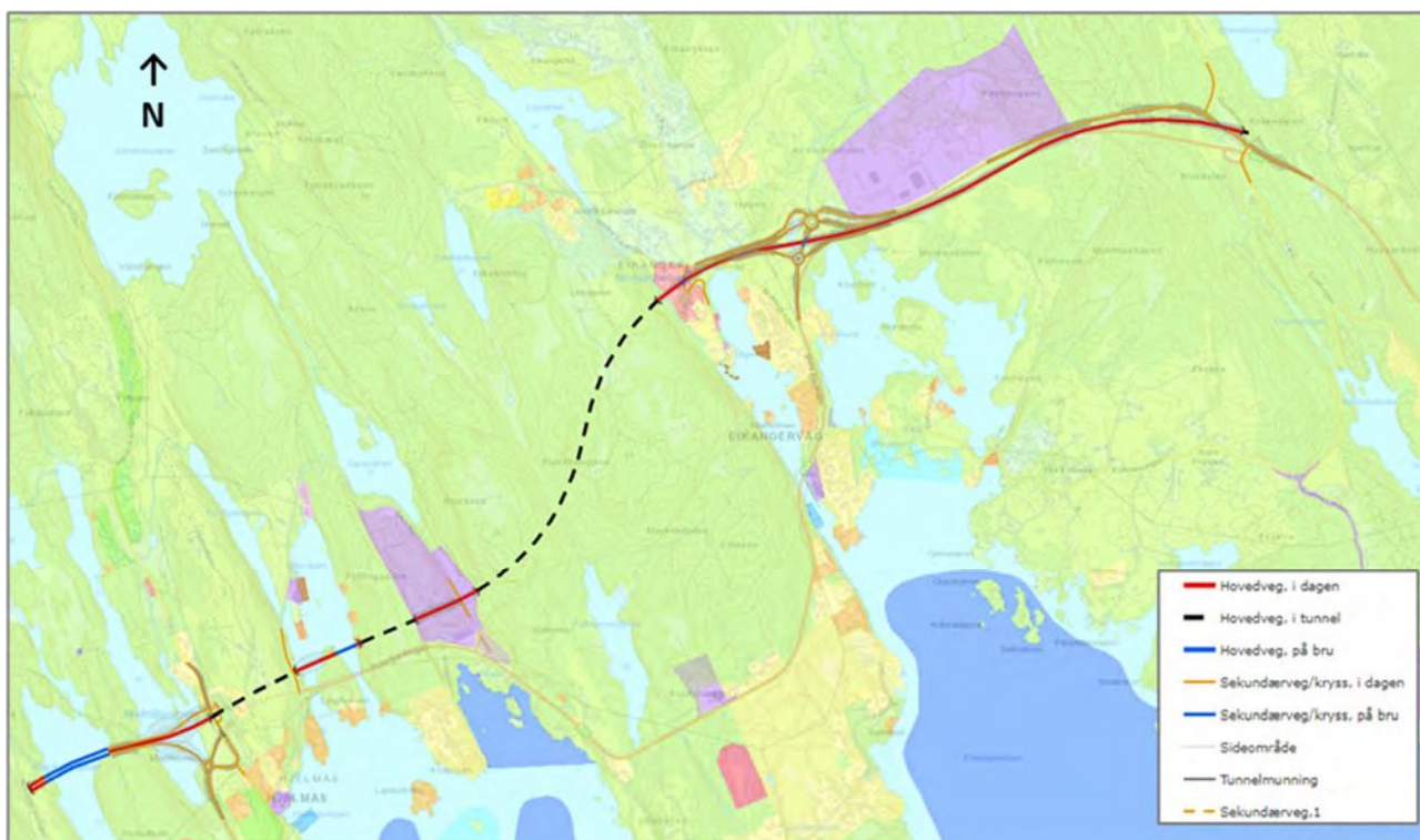
Figur 29. Alternativ M1 vist på arealplan viser kryssing av område avsatt til næringsvirksomhet (lilla skravur) ved Fyllingsnes og ved Kvernhusdalen. Areal for tjenesteyting (rød skravur) ved Eikanger er en skole.
