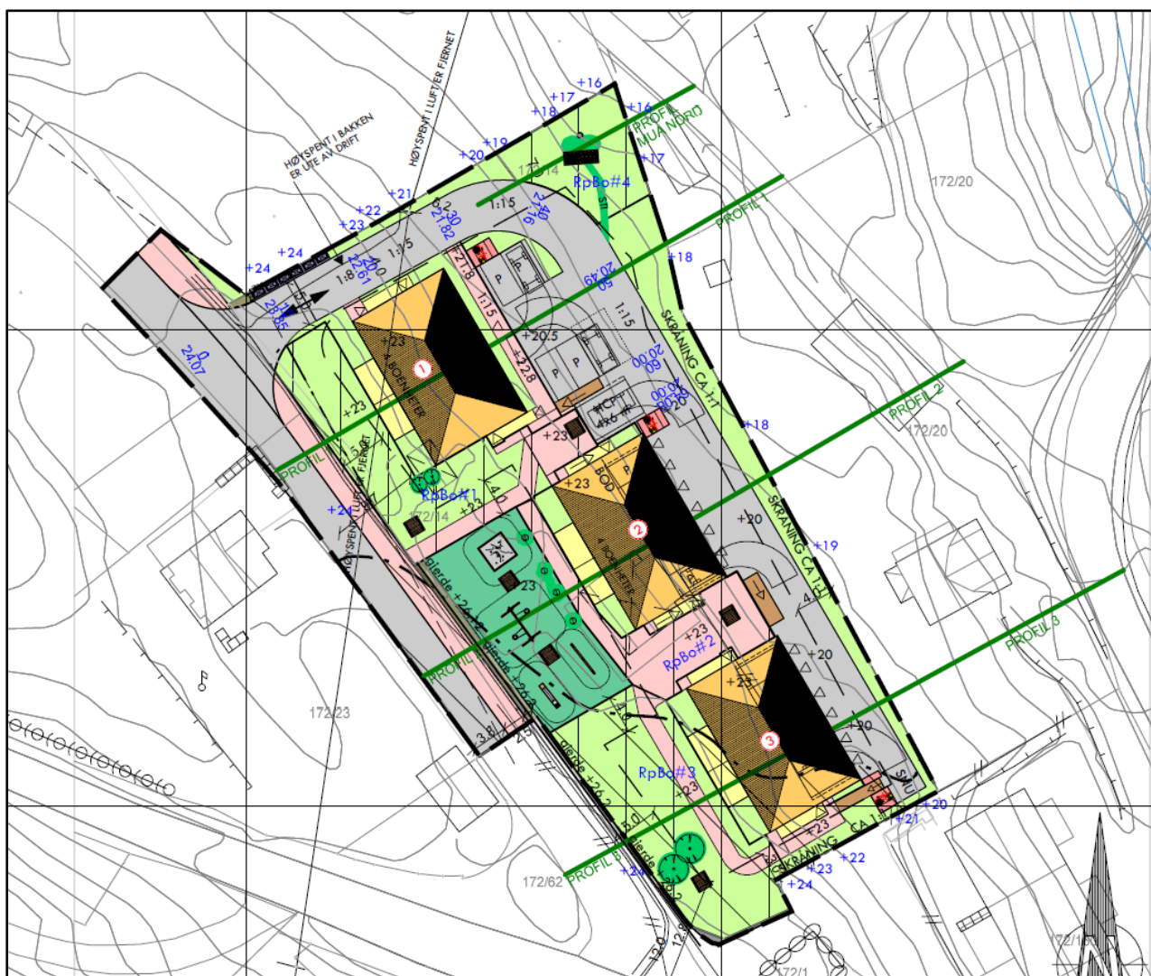
Figur 3-2 Illustrasjonsplan.
