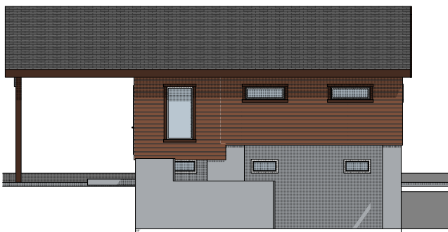
1:200 Fasade Sør
