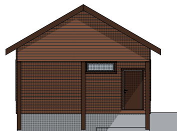
1:200 Fasade Vest
