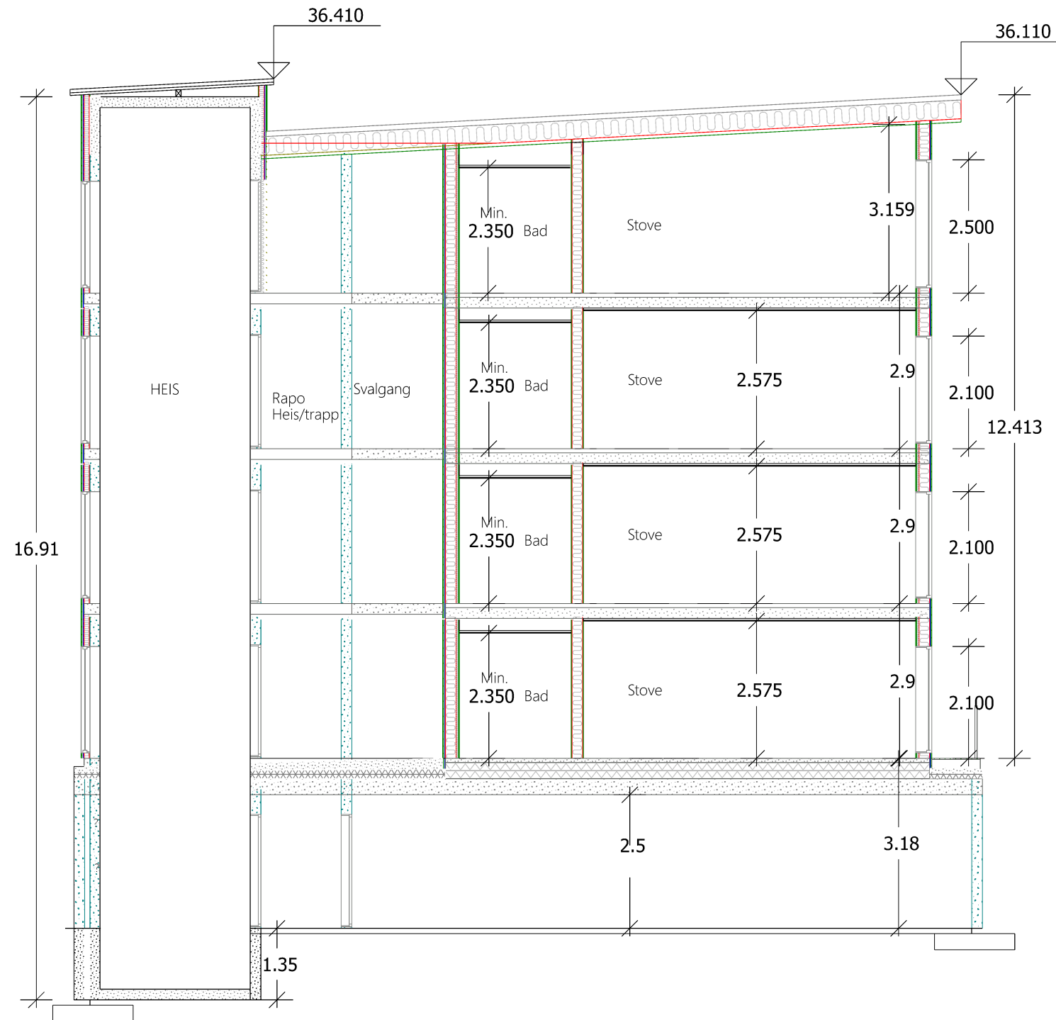
Snitt A-A
