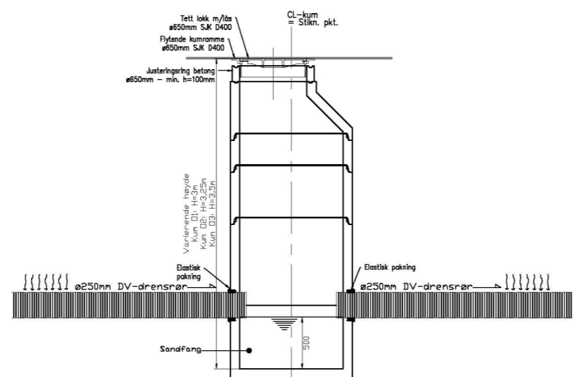
SNITT STAKE-/SANDFANGSKUM O1, O2, O3 M=1:50
