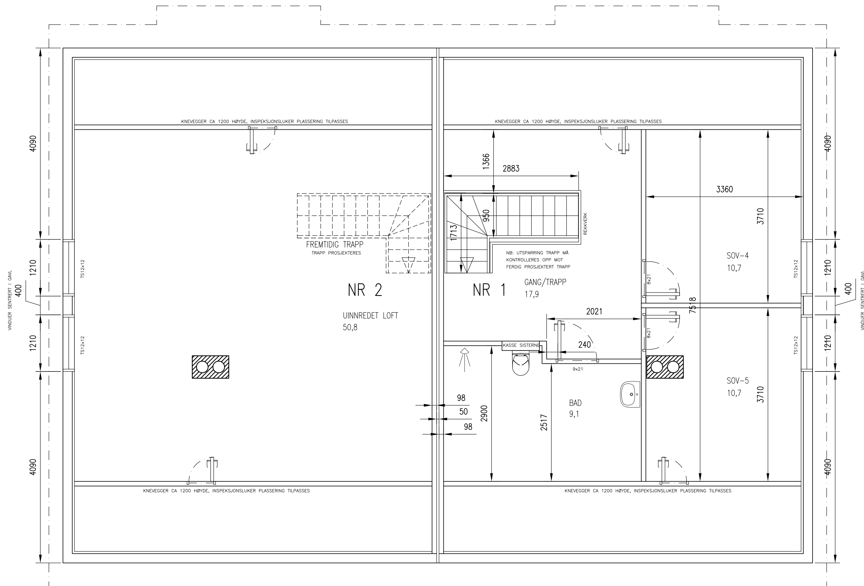
ARBEIDSTEGNING LOFTSPLAN
